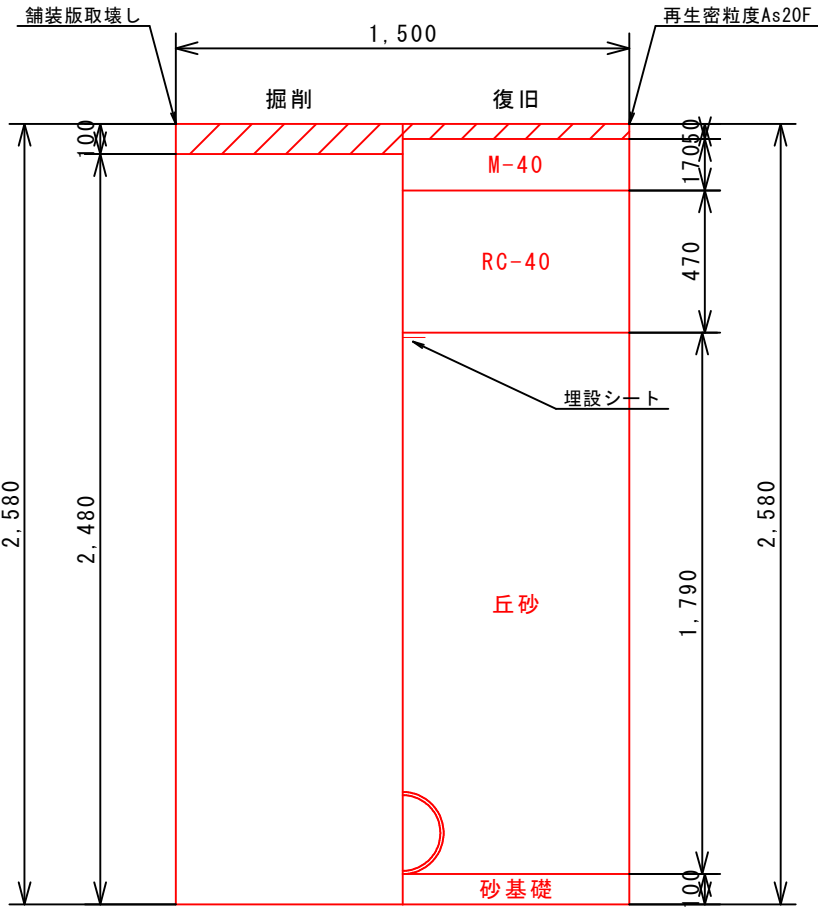
仮復旧断面図 S=1:25
