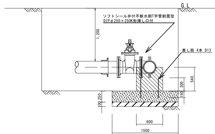
東西断面
