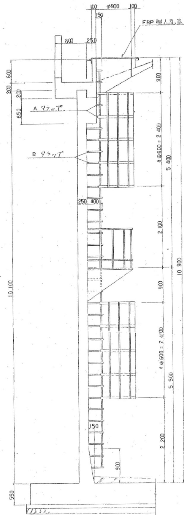
側面図
