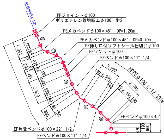
既設管接続工 (1) No. 0+39.540
