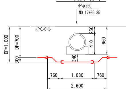
N-N断面図
