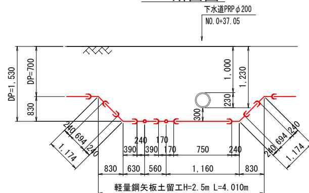
A-A断面図
