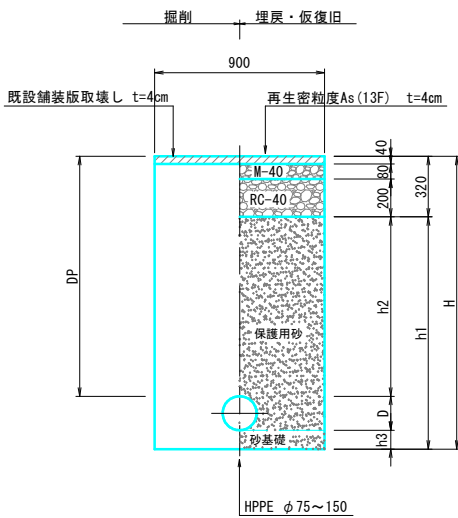
(幹線) ② 市道車道
