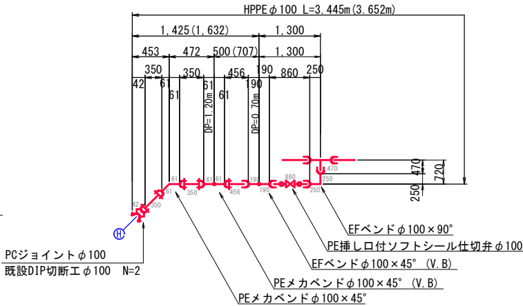
消火栓設置工 (2) No. 0+44.680
