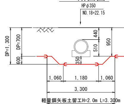
P-P断面図
