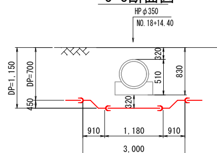
O-O断面図
