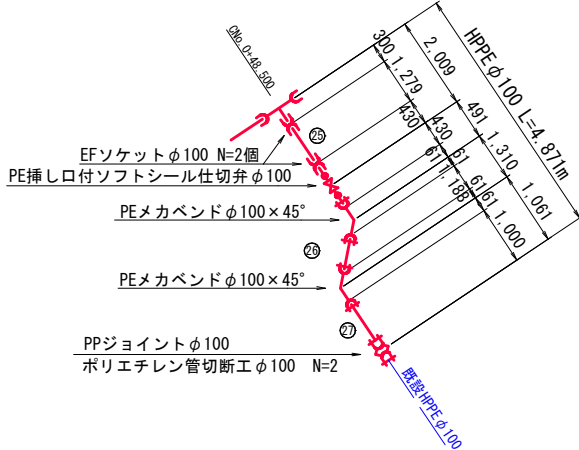
既設管接続工(3)
