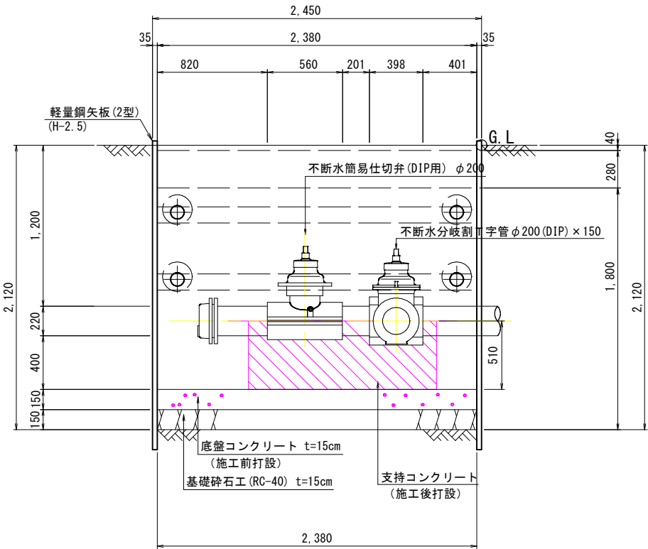
A-A 断面図
