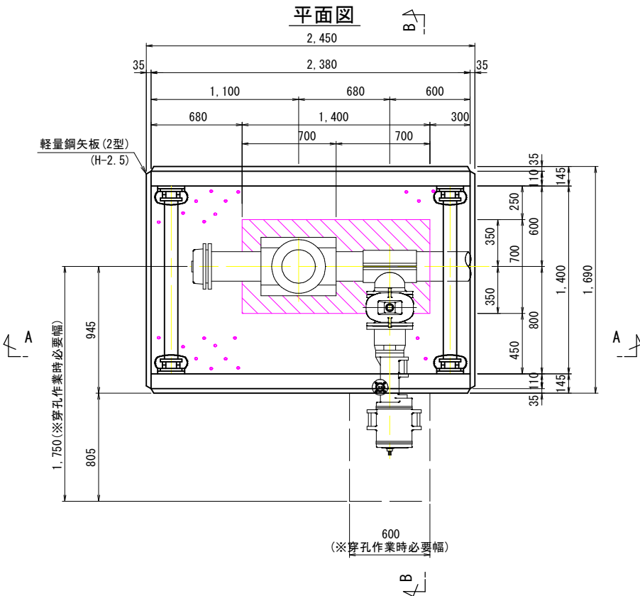
不断水分岐 DIP \phi 200 \times 150 (No. 10+0.980)
