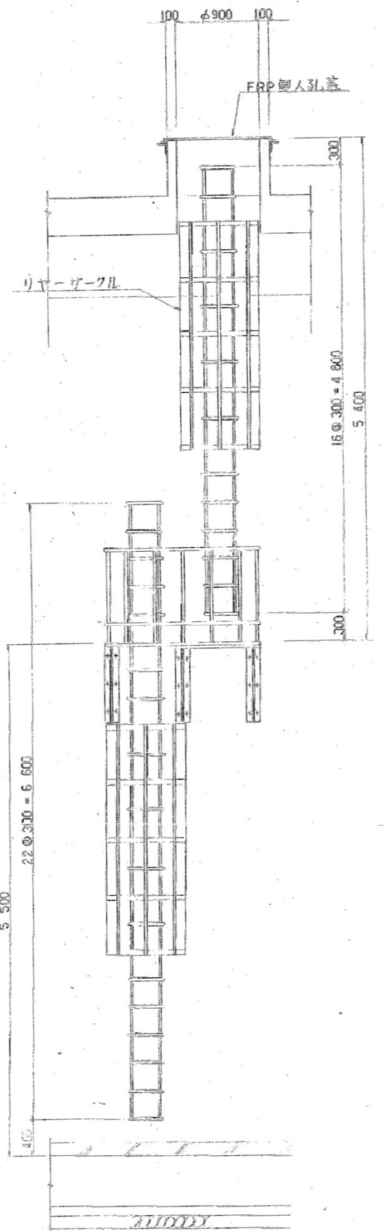
立面図
