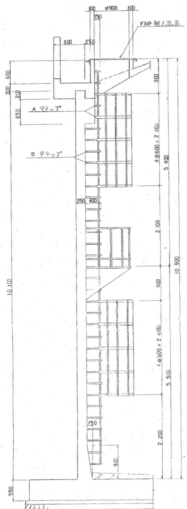
側面図
