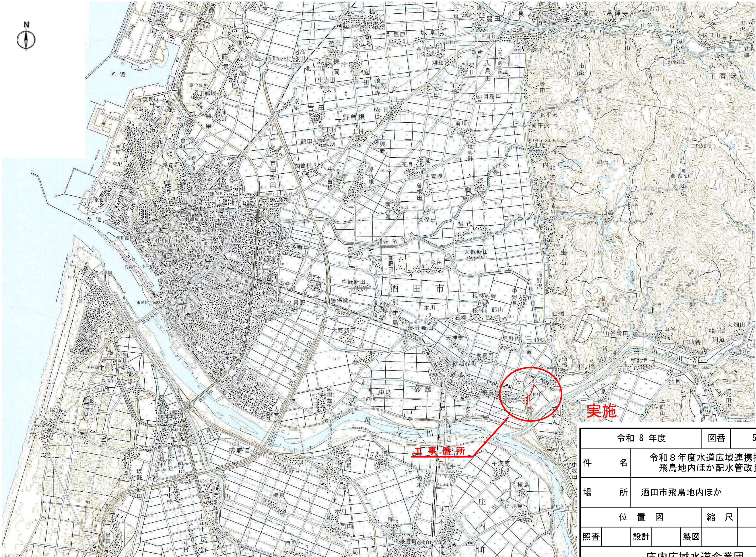
位置図 (縮尺 1/50,000 )
