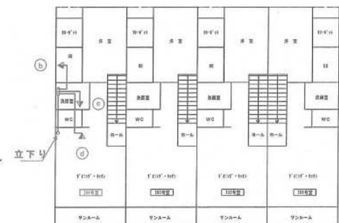
2階給湯平面図
