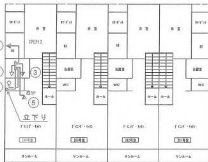
2階給水平面図
