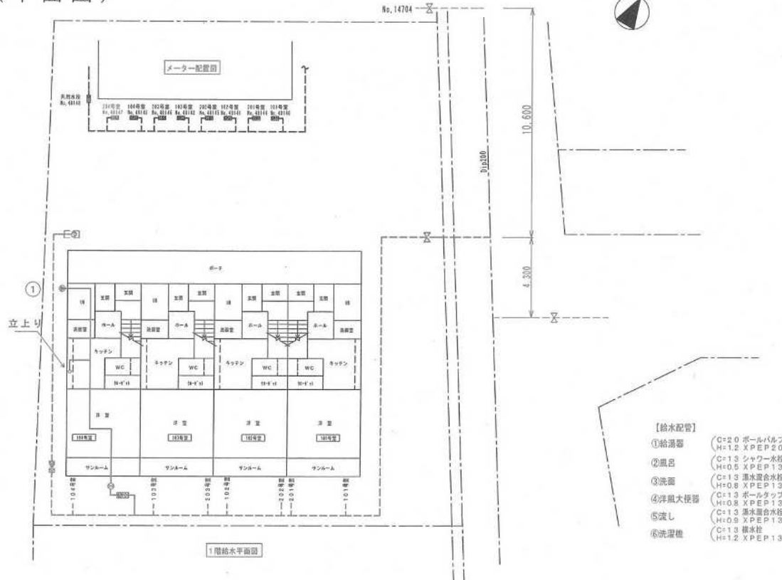
(平面図)
