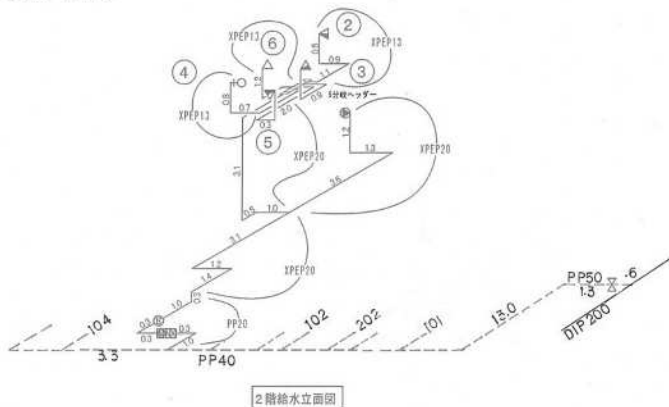
(立面図)
