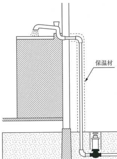
①屋外操作型水抜栓
